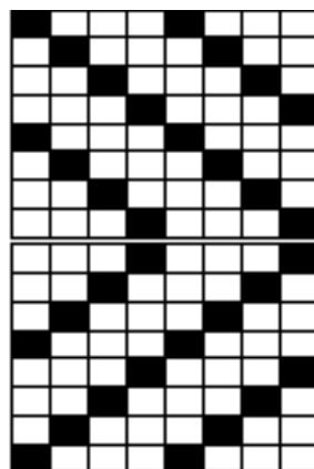
Ligamento sarga de 4
