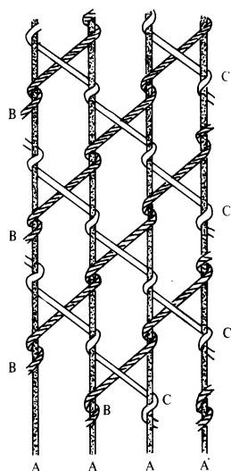
Fig. 1 TUL. A - Hilos de urdimbre. B y C - Hilos de trama oblicuos
