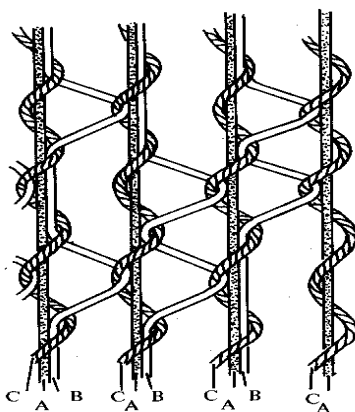
Fig. 3 TUL BOBINOT. A - Hilos de urdimbre. B - Hilos de dibujo. C - Hilos de vuelta.
