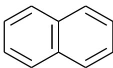
Naftaleno Quinoleína condensada
